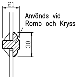
Vertikalsnitt tvärpost
