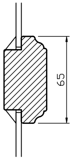
Spröjs
